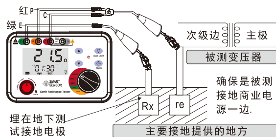
图3：地电阻简易测量
