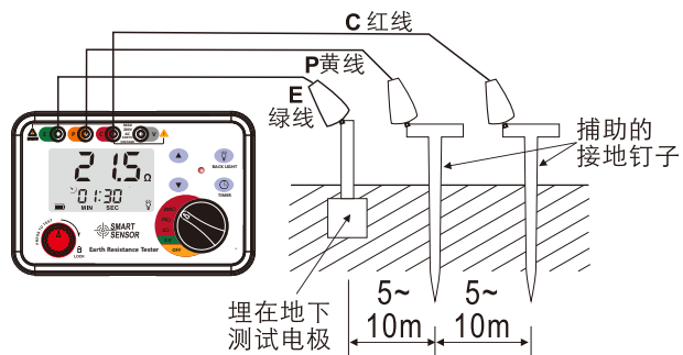
图2：地电阻精确测量
