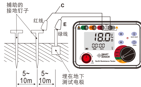
图4：地电压测试图
