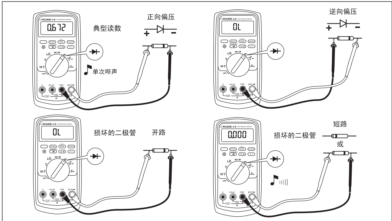
图7. 测试二极管
