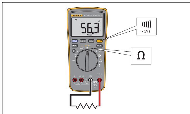
图 3. 测量电阻与通断性
