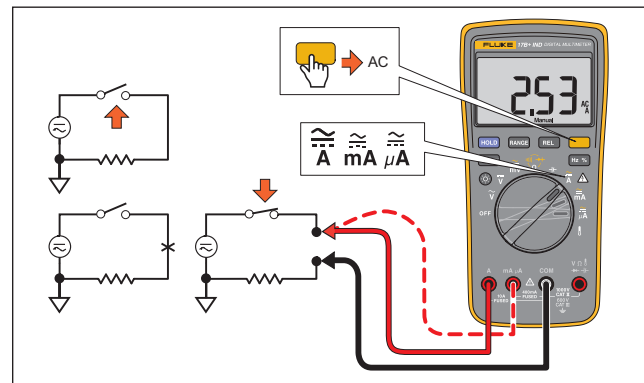
图 2. 测量交流和直流电流
