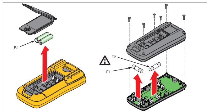
图 4. 更换电池和保险丝
