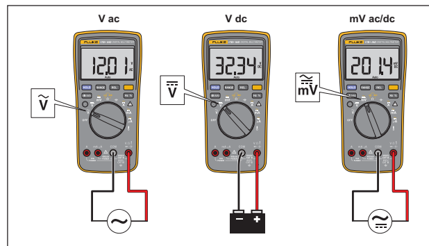
图 1. 测量交流电压和直流电压
