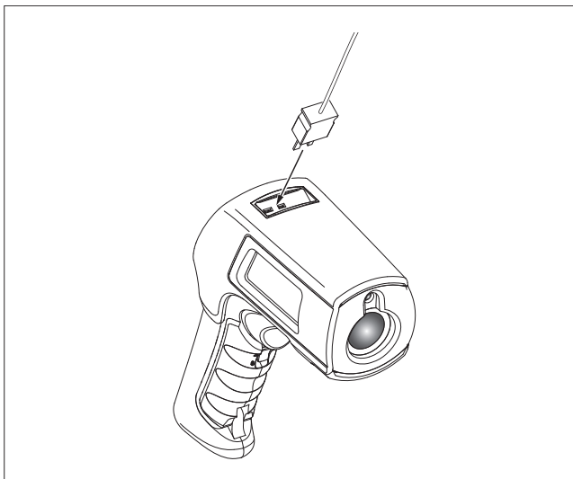
图 7.热电偶连接
